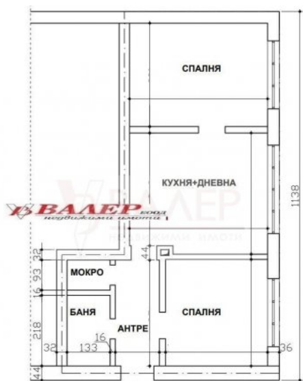
ПЛАН НА АПАРТАМЕНТА М 1:50
